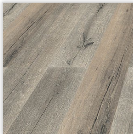
Kolekcja wineo 500 medium V2 , dekor Tirol Oak Silver, symbol LA045MV2. Wymiary [mm]: 1288/195/8. Wzór: pełna deska – rustykalna struktura matowa. Cechy: płyta nośna Aqua Protect, warstwa antystatyczna, klasa ścieralności AC4, montaż bezklejowy LocTec.
